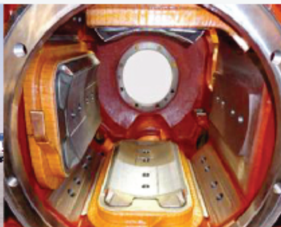
DC MOTOR
